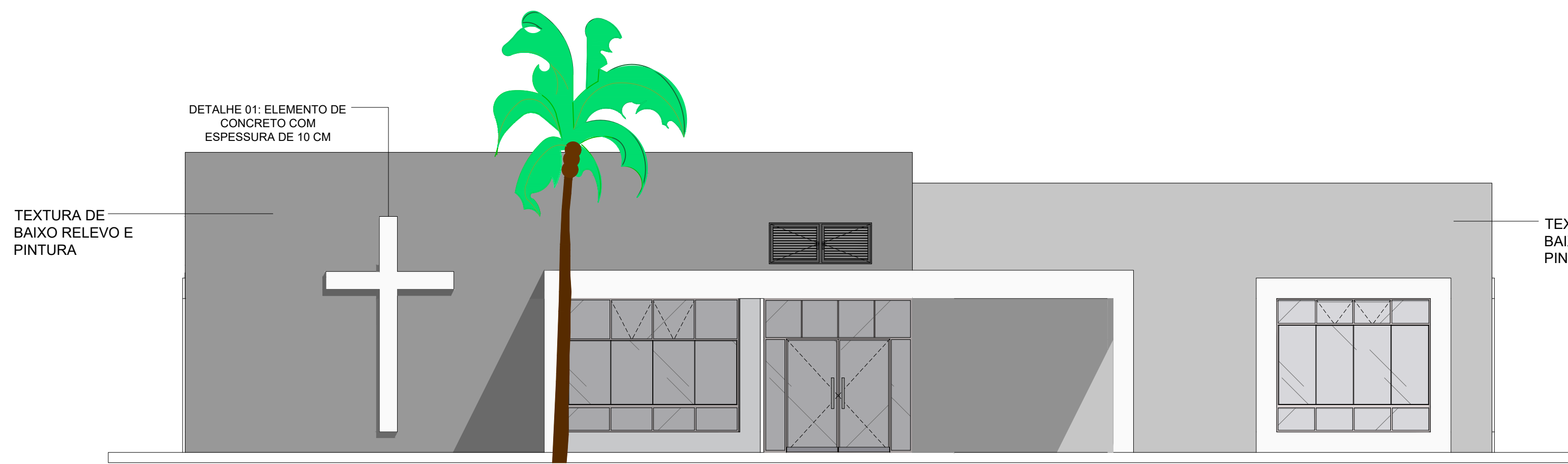
Casa Velatória Fachada SUL ESC: 1/75
