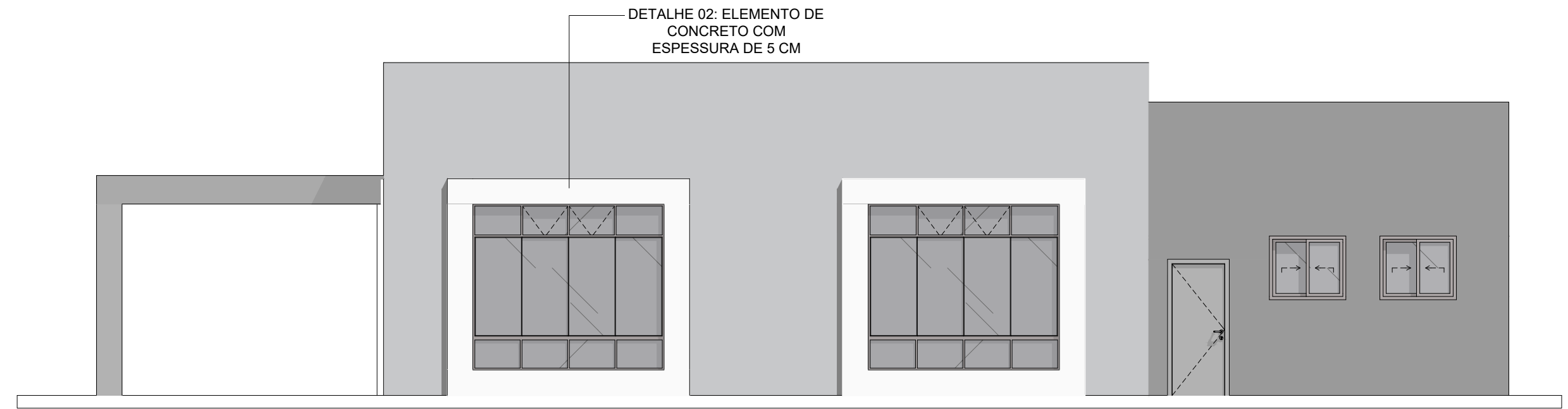
Casa Velatória Fachada LESTE ESC: 1/75
