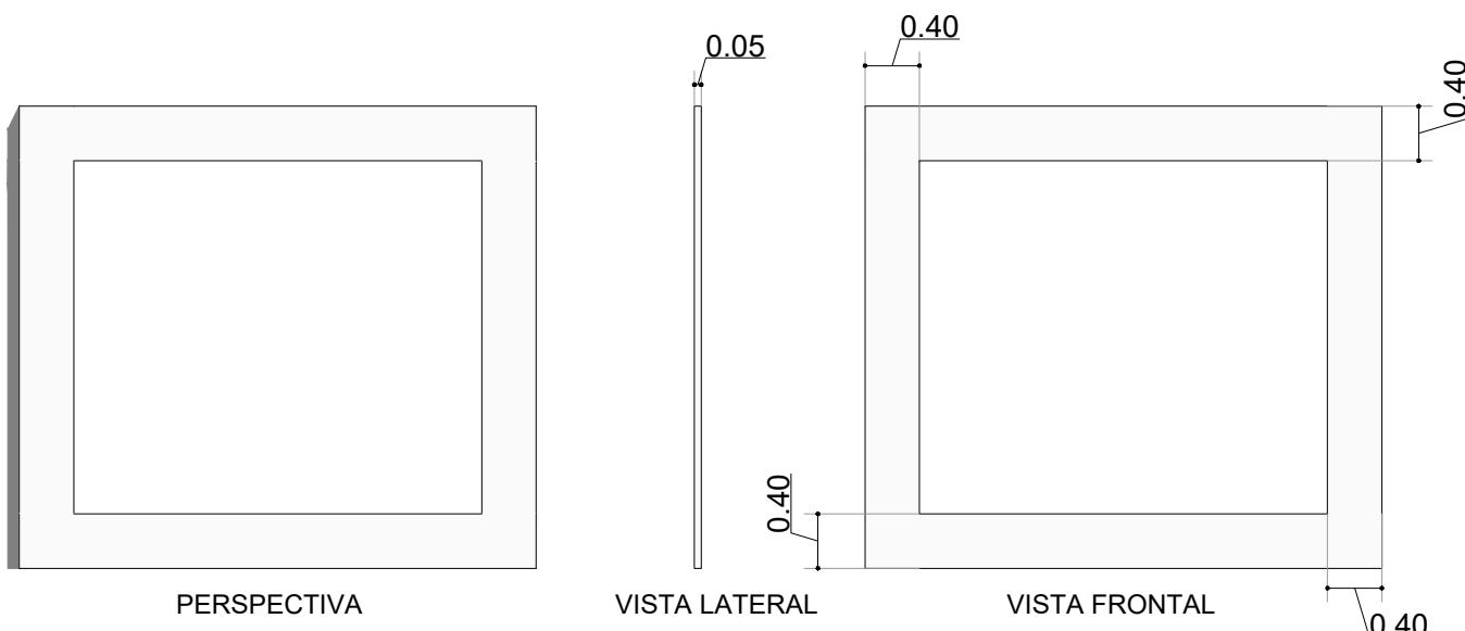
Detalhe 02 - Moldura das janelas
