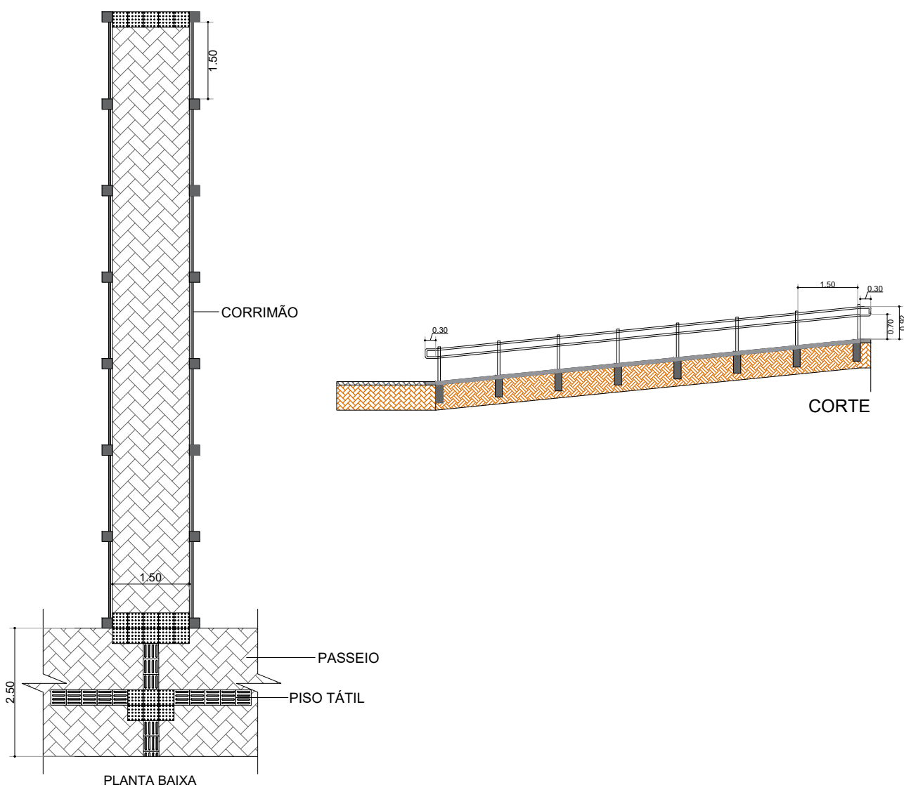
Detalhe 03 - Corrimão e Piso tátil
