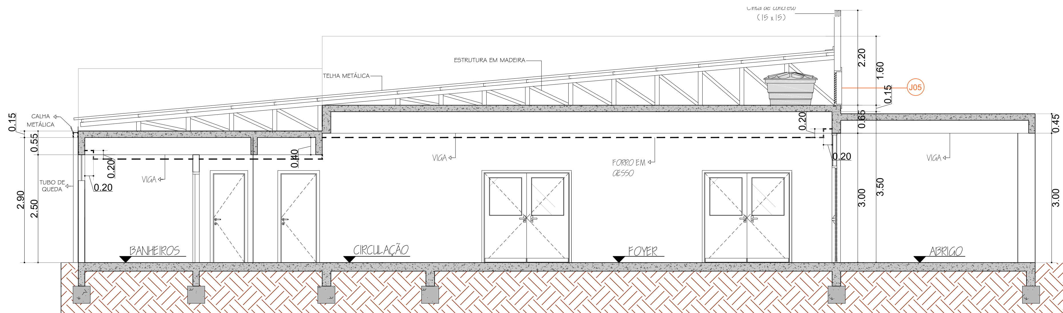
Casa Velatória Corte A-A ESC: 1/100
