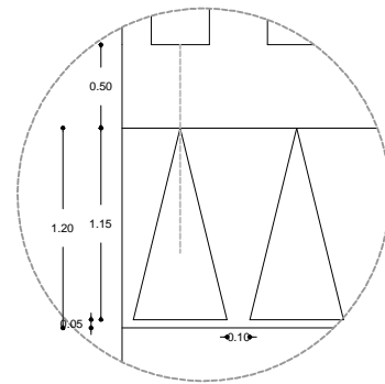
DETALHAMENTO 01 1/20
