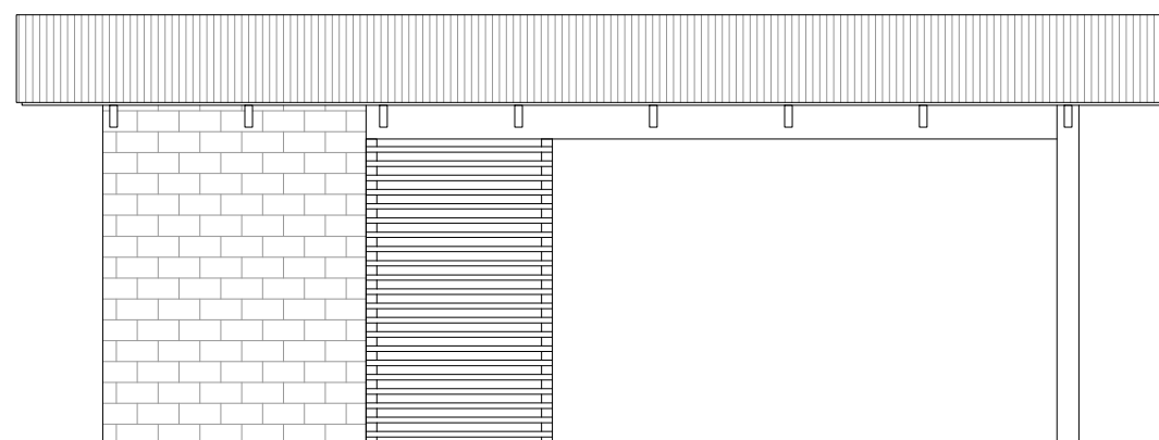
FACHADA SUL
