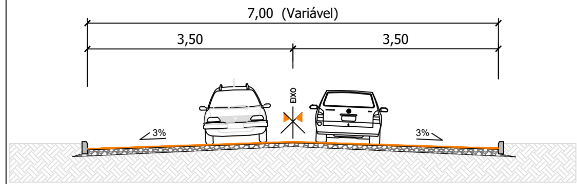
SEÇÃO TIPO Esc.: 1/500 CALÇAMENTO DE PARALELEPÍPEDO COLCHÃO COM PÓ DE PEDRA SUB-LEITO
