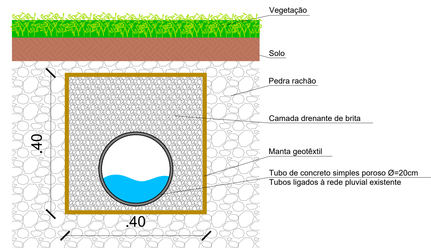
Corte Esc: Sem Escala
